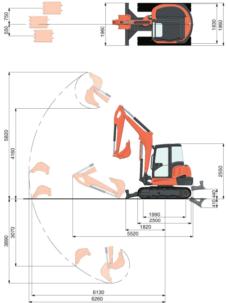
1820 mm langer Löffelstiel Einheit:mm
